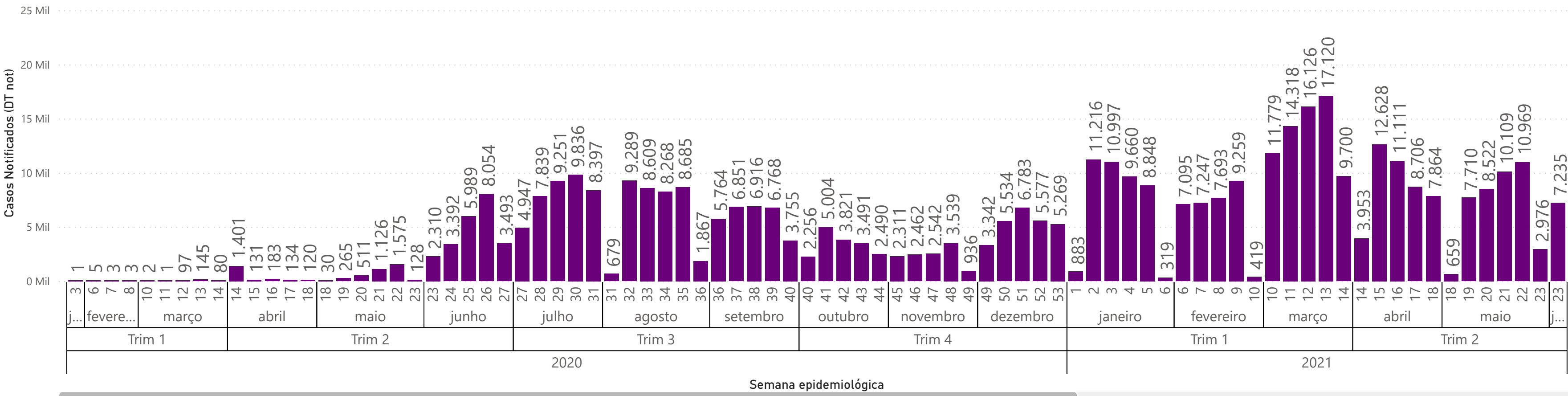
Curva de Casos notificados de COVID-19 por data de notificação em Mato Grosso 2020 2021
